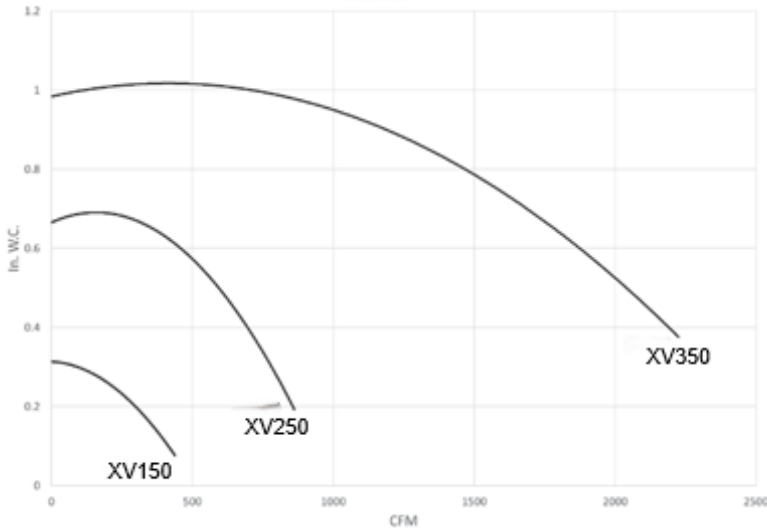
XV FAN CURVES
